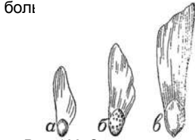
Рис. 106. Семена сосен: а — обыкновенной, б — веймутовой, в — высокой (натуральная величина).
