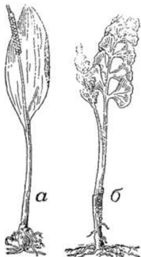
Рис. 100. а — уховник обыкновенный ( Ophioglossum ); б — гроздовик, ключ-трава ( Botrychium ).
